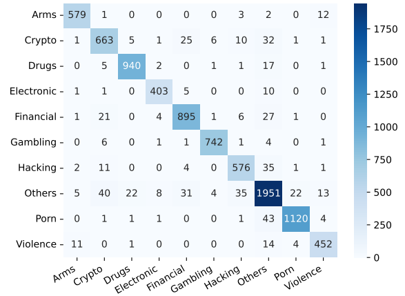
(d) DarkBERT preproc
