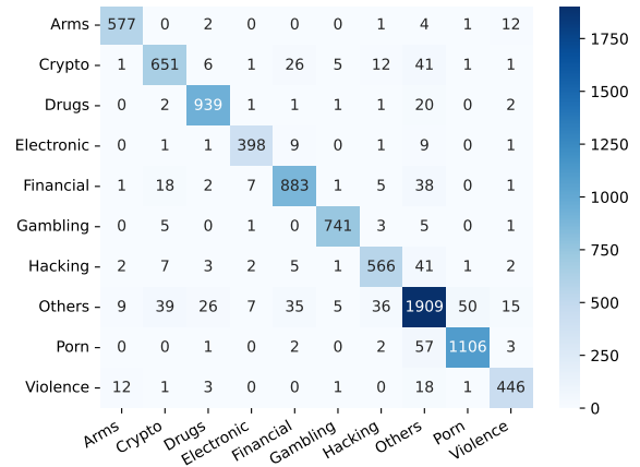
(b) RoBERTa
