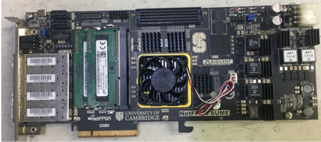
Fig. 6. NetFPGA-SUME.
